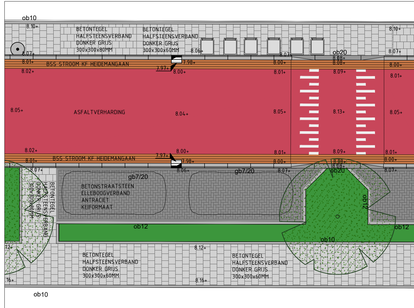
DETAIL 01: BOSLAAN SCHAAL 1:100
