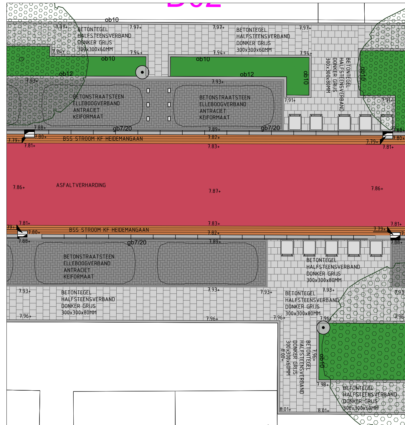
DETAIL 02: BOSLAAN SCHAAL 1:100
